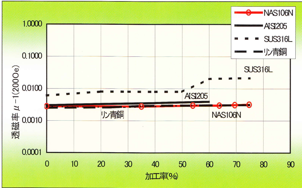
図1 冷間加工率と透磁率の関係 (200Oe)
