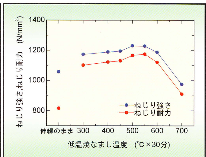
図3 低温焼なましによるねじり特性の変化(φ0.9mmHNF)
