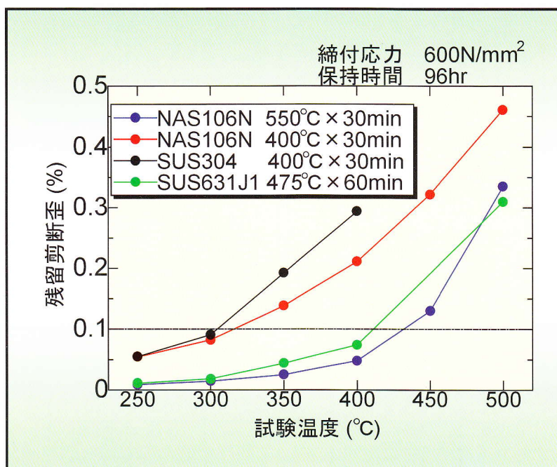
図8 ばねの耐高温へたり特性 ( \Phi 2.0\text{mm} )
