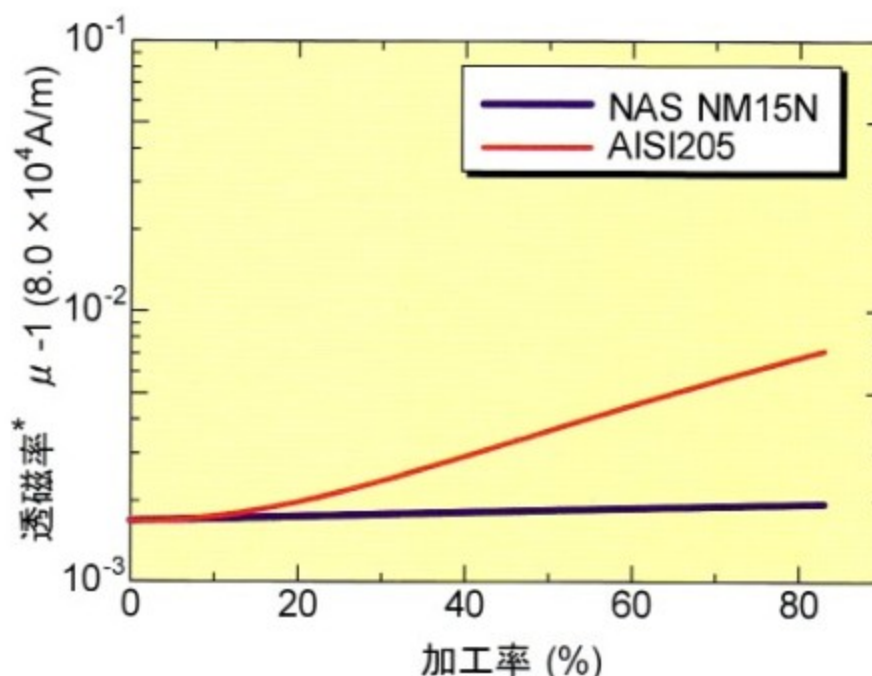
図 3 加工率と透磁率の関係
