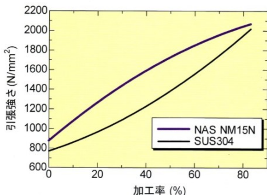
図 2 加工率と引張強さの関係
